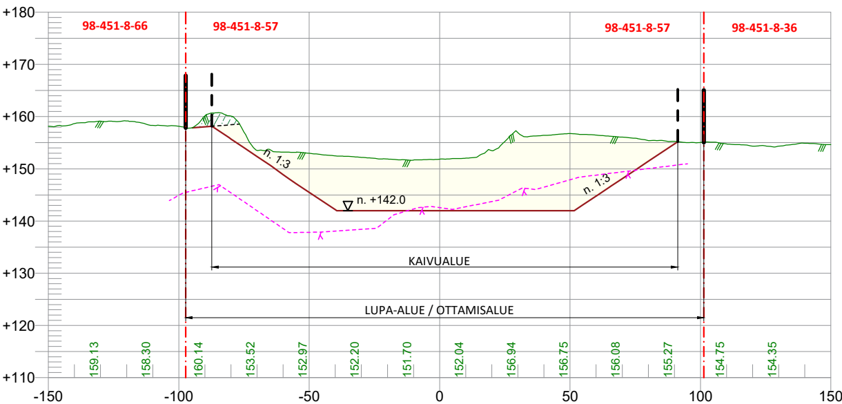
POIKKILEIKKAUS 400-400 1:2000 / 1:1000
