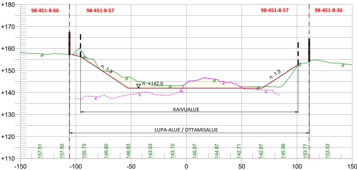
POIKKILEIKKAUS 200-200 1:2000 / 1:1000
