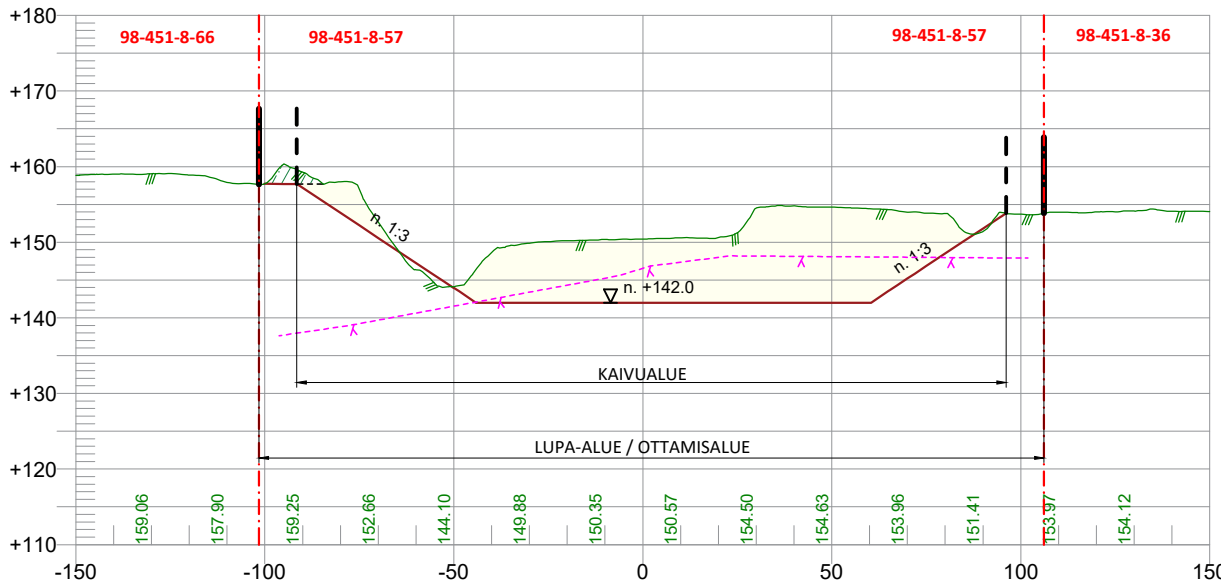
POIKKILEIKKAUS 300-300 1:2000 / 1:1000
