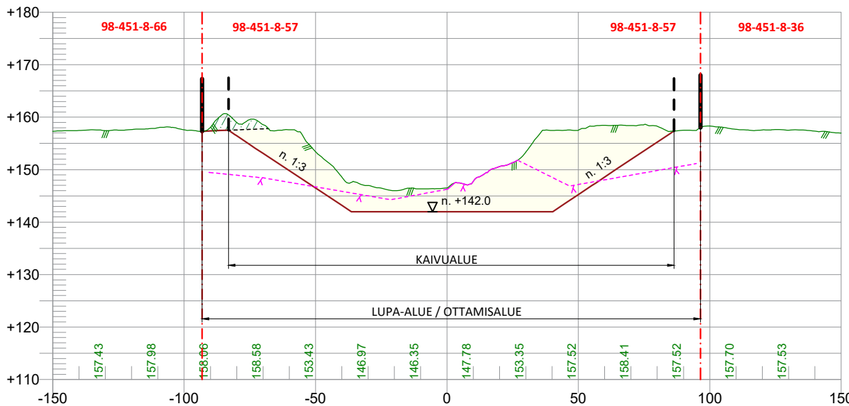
POIKKILEIKKAUS 500-500 1:2000 / 1:1000
